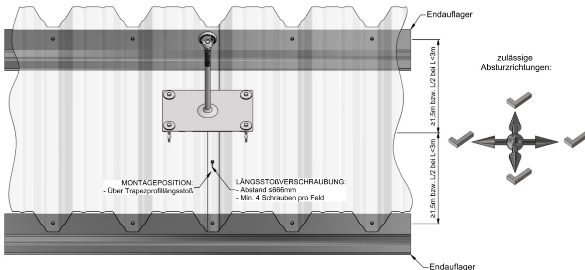
Abbildung 1a - Montagevorgaben auf Trapezprofil (Positivlage) bei Absturzrichtung quer zur Trapezprofilspannrichtung
