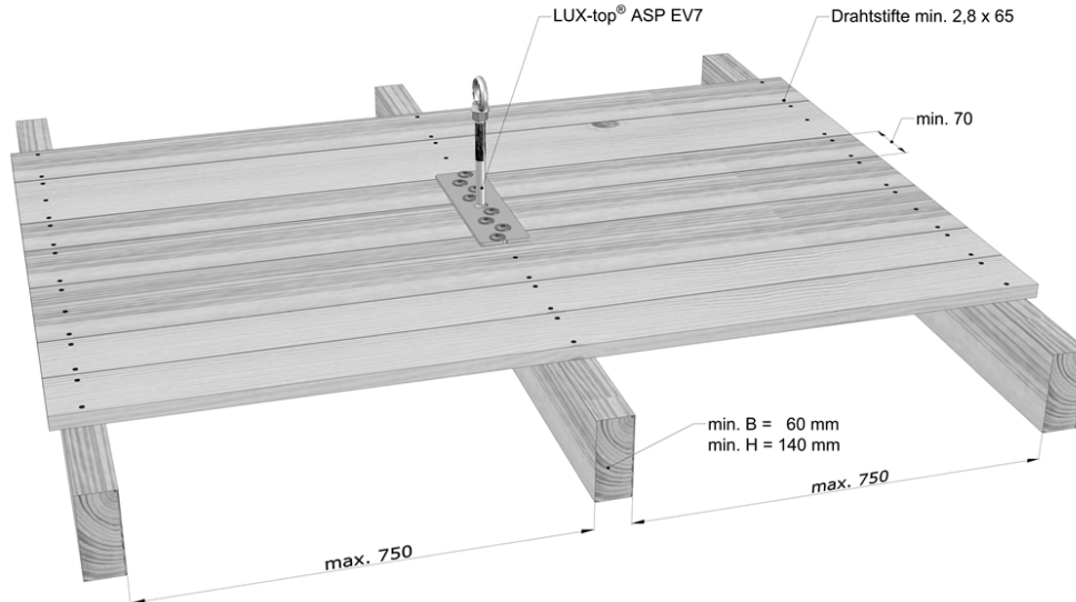
Abbildung 4 - Montagevorgaben - LUX-top® ASP EV 7
