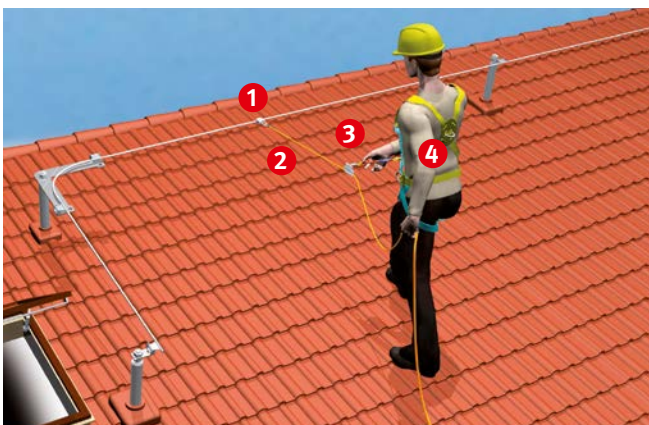
Auffangsystem mit mitlaufendem Auffanggerät einschließlich beweglicher Führung und horizontaler Anschlageinrichtung
