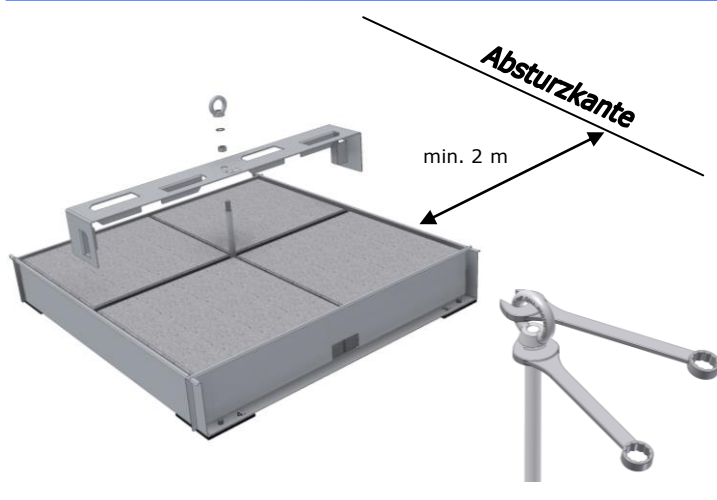
Abb. 10: Montage der Lastverteilplatte u. Sichern der Anschlagöse
