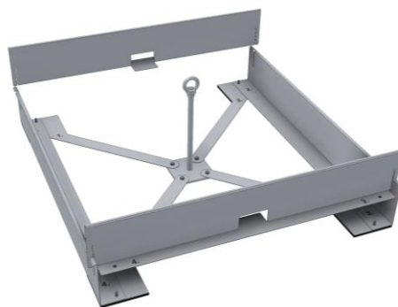
Figure 5 : emboîtement des parties latérales supérieures
