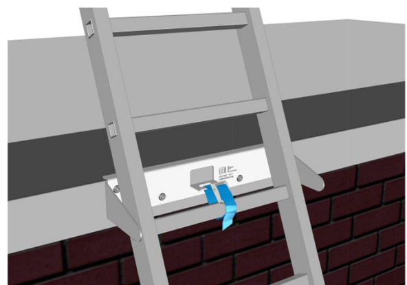
Abb. 2: LUX-top® LS I mit gesicherter Anlegeleiter
