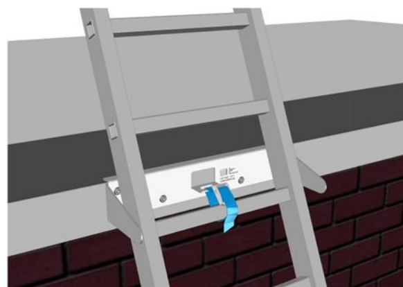
Image 2 : LUX-top® LS I avec échelle simple sécurisée
