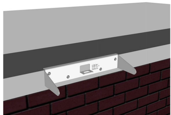
Abb. 1: LUX-top® LS I montiert am Attikablech
