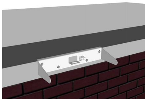
Image 1 : LUX-top® LS I fixé sur recouvrement de l'acrotère
